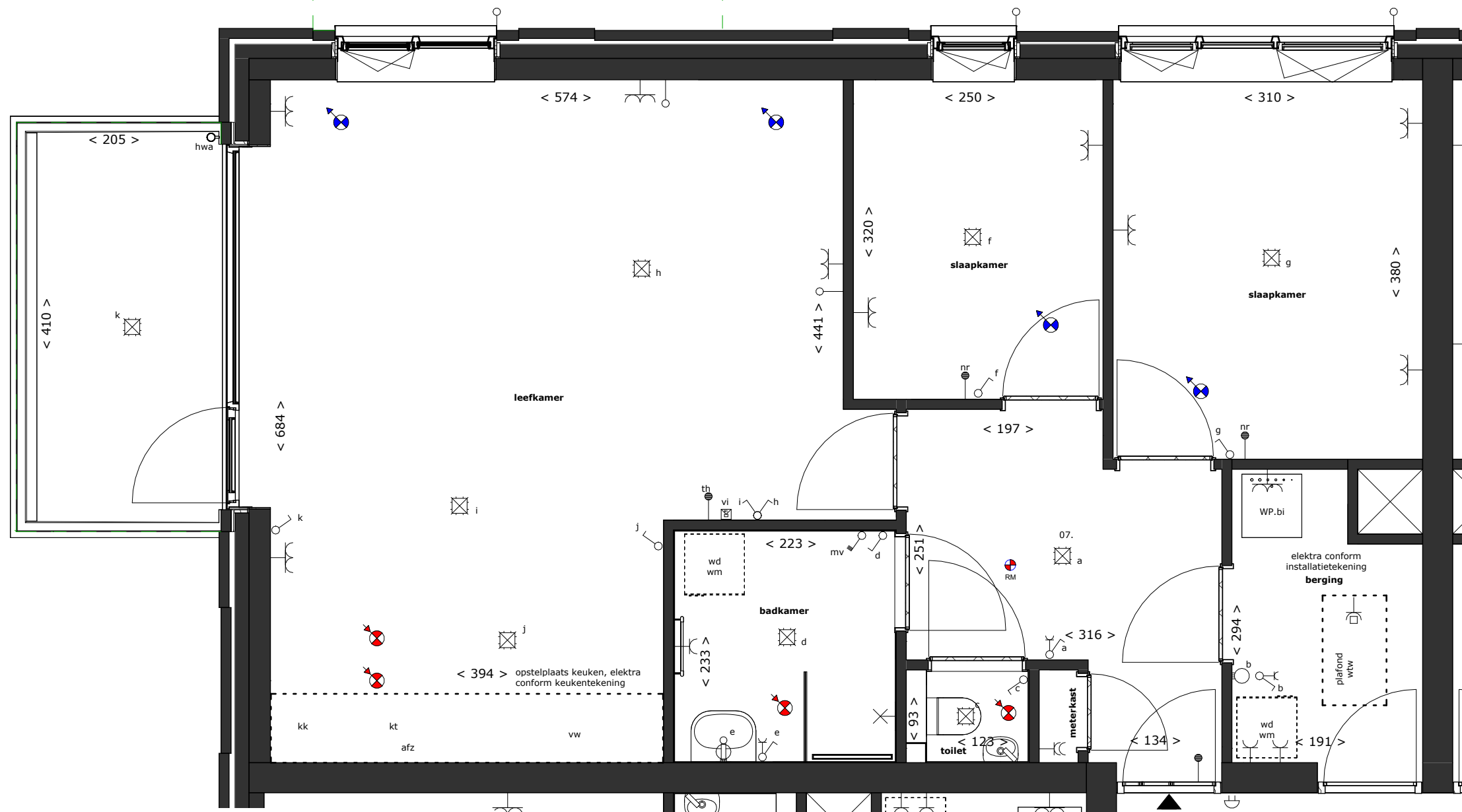
v.01. eerste verdieping - bouwnummer 7
