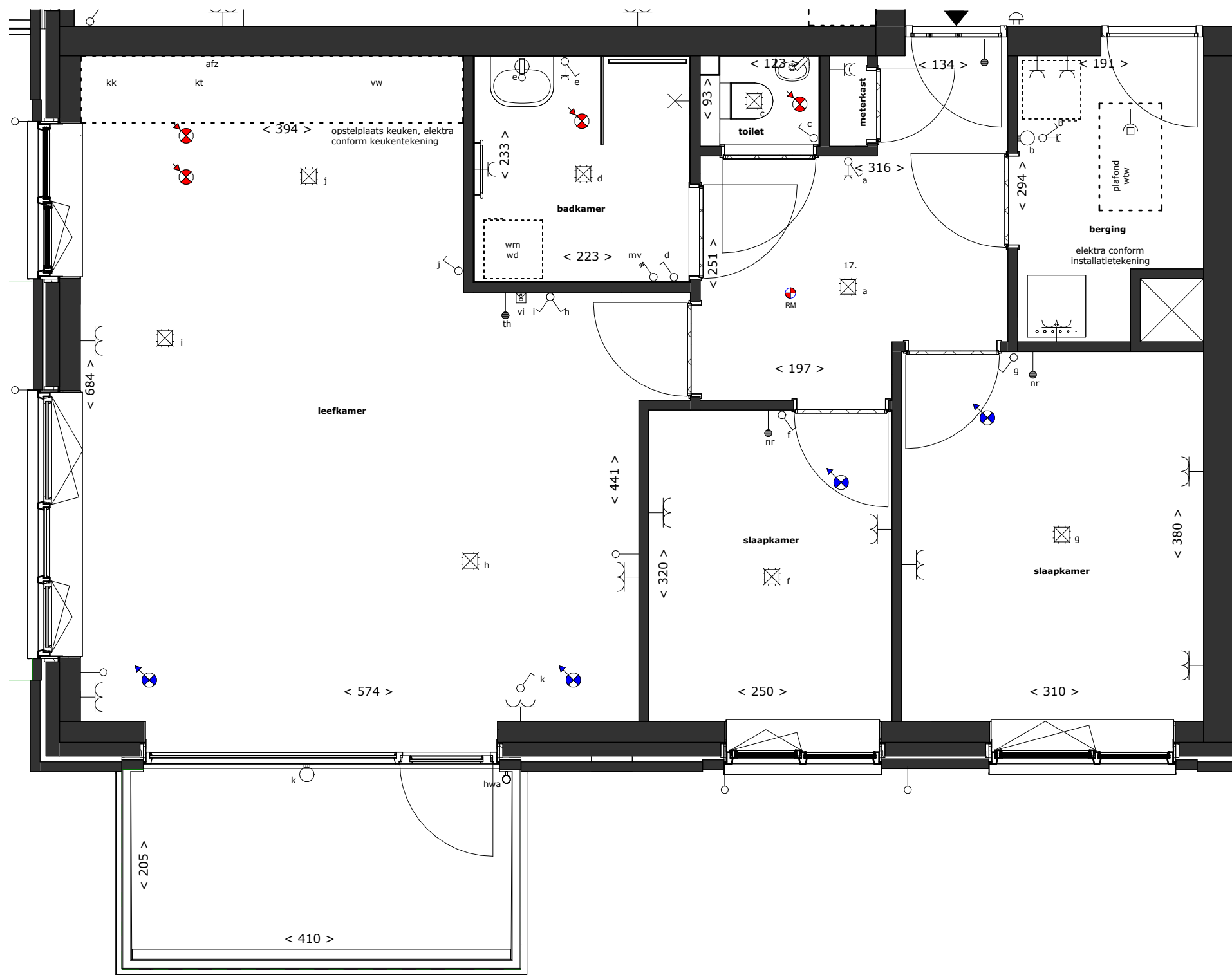
v.03. derde verdieping - bouwnummer 17 1 : 50
