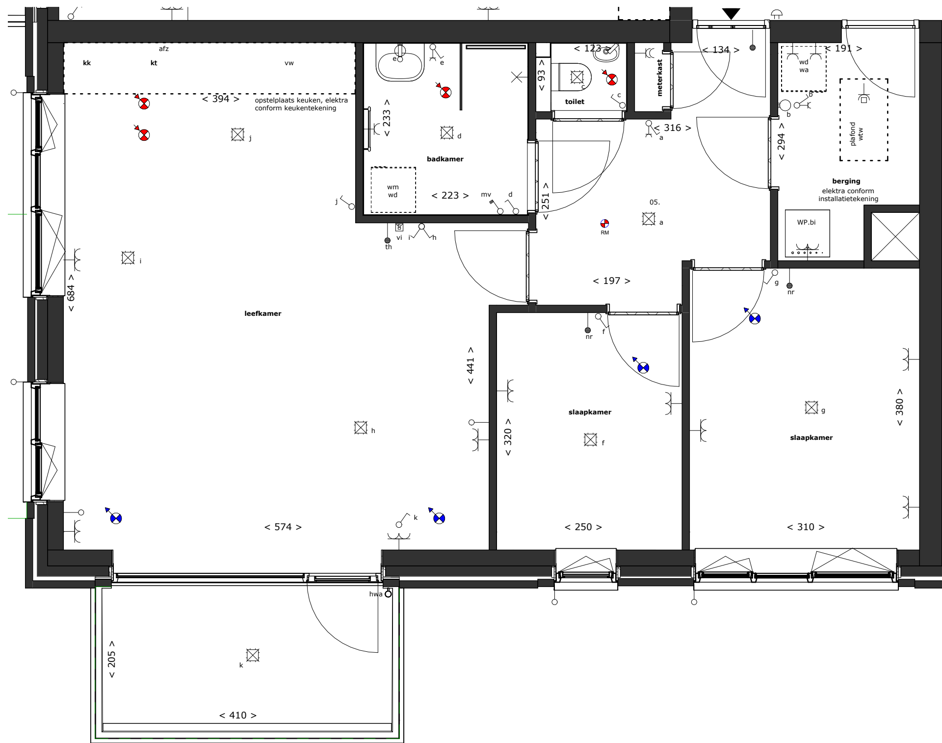
v.01. eerste verdieping - bouwnummer 5 1 : 50
